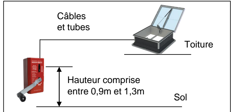
Treuil BT 130
