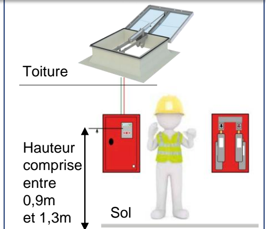
Boitier Dioxy Désenfumage pneumatique et aération
